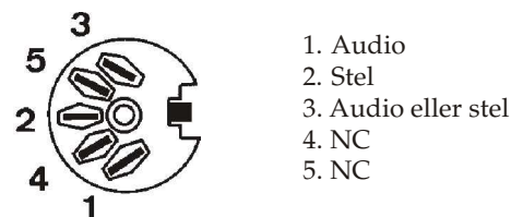
Fig. 2 Audio indgangsbøsning set fra bagsiden af modulatoren
